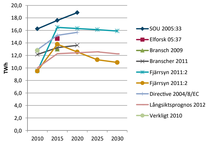
Figur 1: Sammanställning av ett antal tidigare potentialbedömning av elproduktionen i kraftvärmeverk i svenska fjärrvärmesystem.
