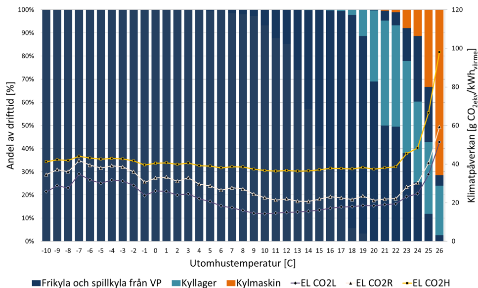
Figur 4.9: Temperaturindelat marginalmix (vänster Y-axel) för fjärrkylenät emissionsvektorer (höger Y-axel) för tre elscenarier. Staplarna anger en fördelning för hur en trolig marginalmix ser ut vid en viss utomhustemperatur. Emissionsvektorn anger CO 2e -emissionerna som är kopplad till samma marginalmix och utomhustemperatur. Grafen är framtagen i enlighet med metodsteg 5-6 i Figur 4.1. Scenariobeteckningar: L – Låg, H – Hög (för vidare scenaroförklaring, se avsnitt 5.2).
