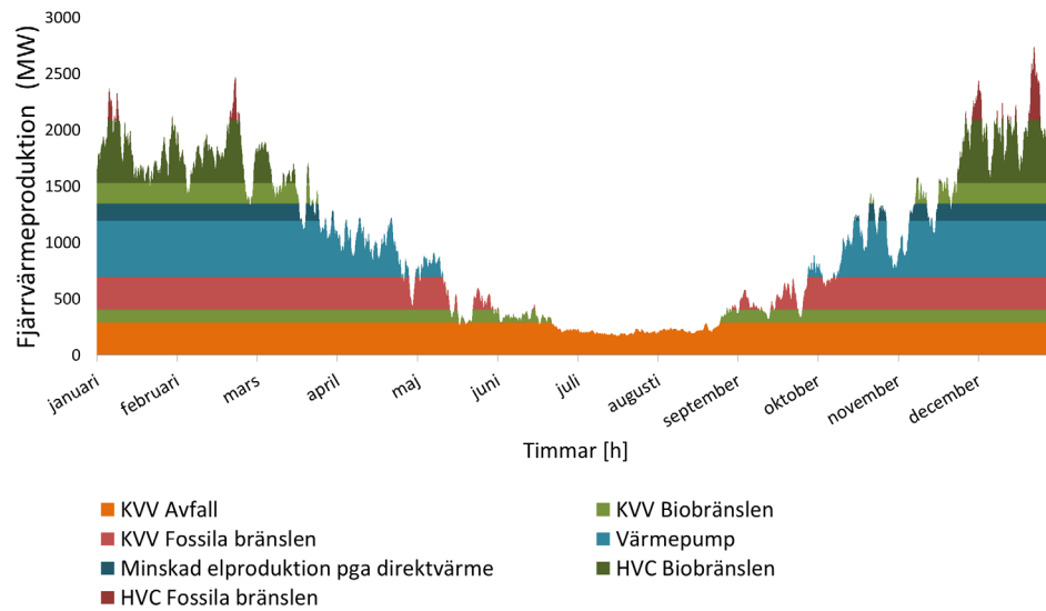
Figur 4.2: Simulerad fjärrvärmeproduktion (8760 timmar) för stort typnät enligt metodsteg 1-4 i Figur 4.1. (KVV, kraftvärme; HVC, hetvattencentral)
