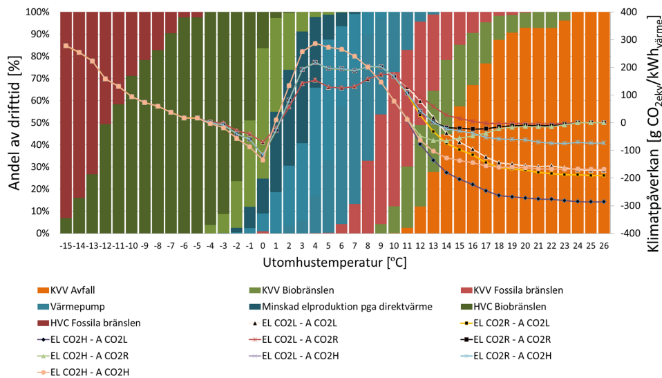
Figur 4.3: Temperaturindeldad marginalmix (vänster Y-axel) för stort nät samt fjärrvärmenätets emissionsvektor (höger Y-axel) för tre elscenarier och tre avfallsscenarier. Staplarna anger en fördelning för hur en trolig marginalmix ser ut vid en viss utomhustemperatur. Emissionsvektorn anger CO 2e -emissionerna som är kopplad till samma marginalmix och utomhustemperatur. Grafen är framtagen i enlighet med metodsteg 5-6 i Figur 4.1. Scenariobeteckningar: L – Låg, R – Referens, H – Hög, A – Avfall (för vidare scenaroförklaring, se avsnitt 5.2 och 6.2).
