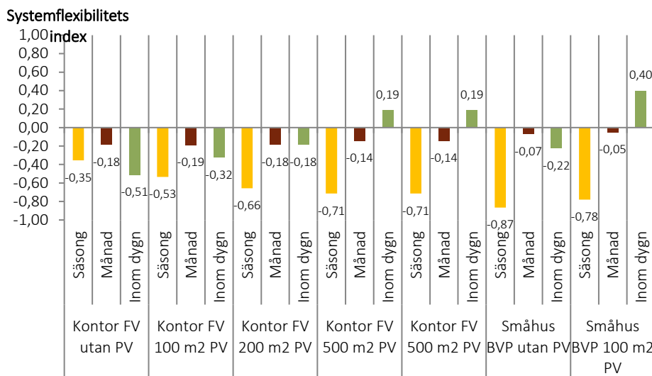
Figur E.1 Exempel på systemflexibilitetsindex. Positiva värden innebär att byggnadens elförbrukning har en positiv korrelation till icke planerbar produktion, vilket innebär att planerbar kraft frigörs. Ett negativ värde innebär att byggnaden har en hög förbrukning av el när andelen icke planerbar kraft i systemet är lågt, vilket ger ett högt behov av planerbar kraft. (FV, fjärrvärme; PV, solceller; BVP, bergvärmepump)
