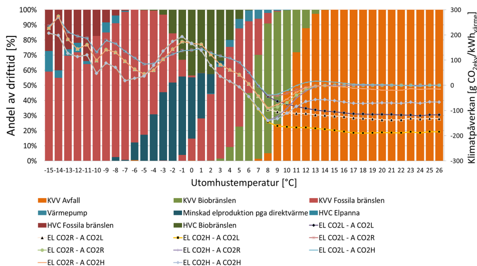
Figur 4.5: Temperaturindeldad marginalmix (vänster Y-axel) för medelstort nät samt fjärrvärmenätets emissionsvektor (höger Y-axel) för tre elscenarier och tre avfallsscenarier. Staplarna anger en fördelning för hur en trolig marginalmix ser ut vid en viss utomhustemperatur. Emissionsvektorn anger \text{CO}_{2e} -emissionerna som är kopplad till samma marginalmix och utomhustemperatur. Grafen är framtagen i enlighet med metodsteg 5-6 i Figur 4.1. Scenariobeteckningar: L – Låg, R – Referens, H – Hög, A – Avfall (för vidare scenaroförklaring, se avsnitt 5.2 och 6.2).
