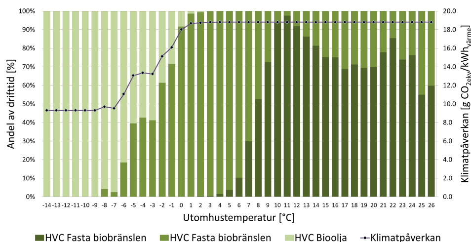
Figur 4.7: Temperaturindeldad marginalmix (vänster Y-axel) för litet nät samt fjärrvärmenätets emissionsvektor (höger Y-axel). Staplarna anger en fördelning för hur en trolig marginalmix ser ut vid en viss utomhustemperatur. Emissionsvektorn anger CO 2e -emissionerna som är kopplad till samma marginalmix och utomhustemperatur. Grafen är framtagen i enlighet med metodsteg 5-6 i Figur 4.1.
