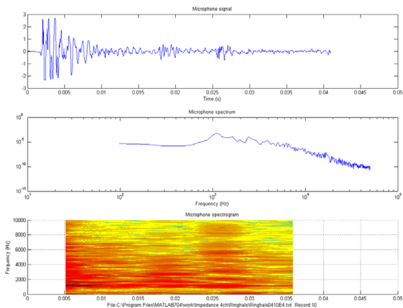
Figur 4 Slag med snickarhammare samt inspelning av ljudsignal från stationär mikrofon. Mätningen triggas igång av ljudpulsen från slaget. Den akustiska bakgrunds-nivån, som framgår av de första 2 ms data, ligger som synes långt under signalnivån från slaget. Ingen kraftsignal registreras och snickarhammaren behöver inte ha någon förbindelse med mätutrustningen.
