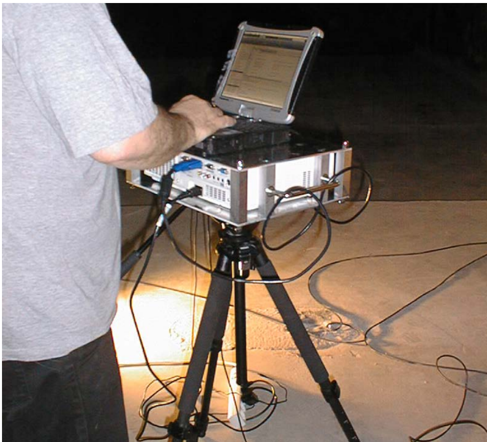
Figur B 6 Närbild på dator och projektor inbyggd i skyddskåpa.
