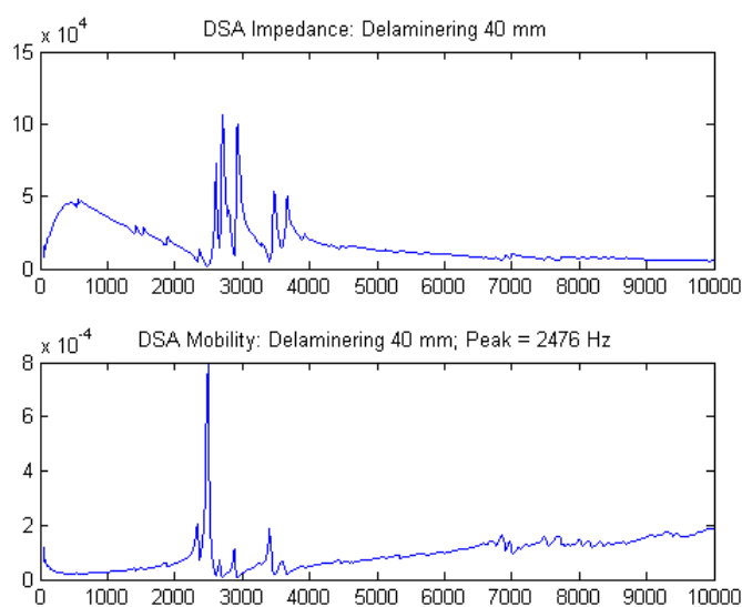
Figur 1 Impedans och motsvarande mobilitet uppmätt genom frekvensvep.
