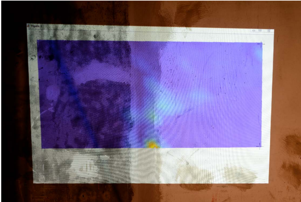
Figur B 11 Denna bild visar det interpolerade resultatet av undersökningen med hammare och geofon projicerat på mätytan. Genom att jämföra denna bild med en bild som markerar mätområdets kant, kan man lokalisera läget för skadade partier relativt visuella markers på ytan. Man kan också rita av de skadade partierna på mätytan direkt.
