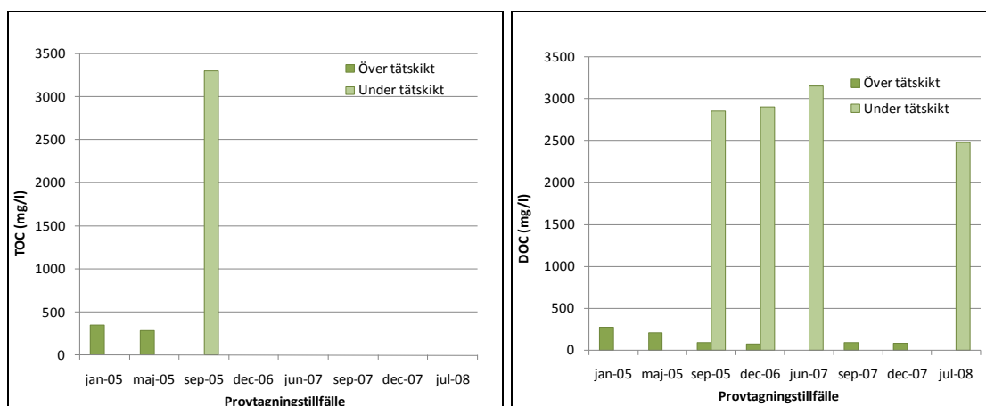
Figur 2-5 Halter organiskt kol (totalt respektive löst) i vatten från lysimetrar och avrinningsytor i provytan på Gärstad. Medelvärde har beräknats för provtagningspunkter över respektive under tätskiktet.
