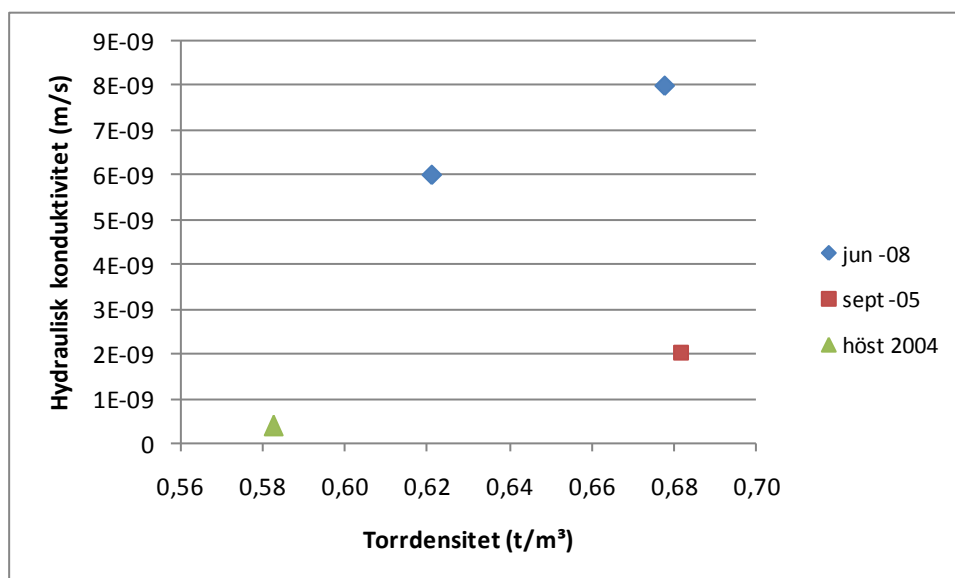
Figur 2-13 Hydraulisk konduktivitet jämfört med densitet för prover av FSA från Gärsstad.
