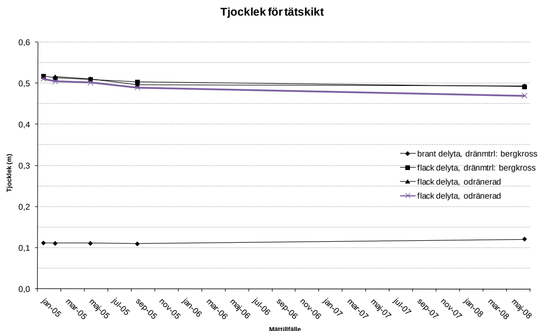
Figur 2-10 Tjocklek för tätskikt vid sättningspegel på olika delytor, Gärstad.
