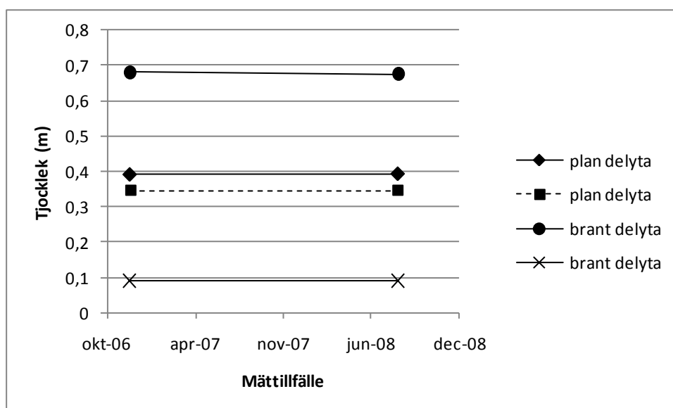
Figur 2-9 Tjocklek för tätskiktet vid sättningspegelarna på olika delytor, Sofielund.
