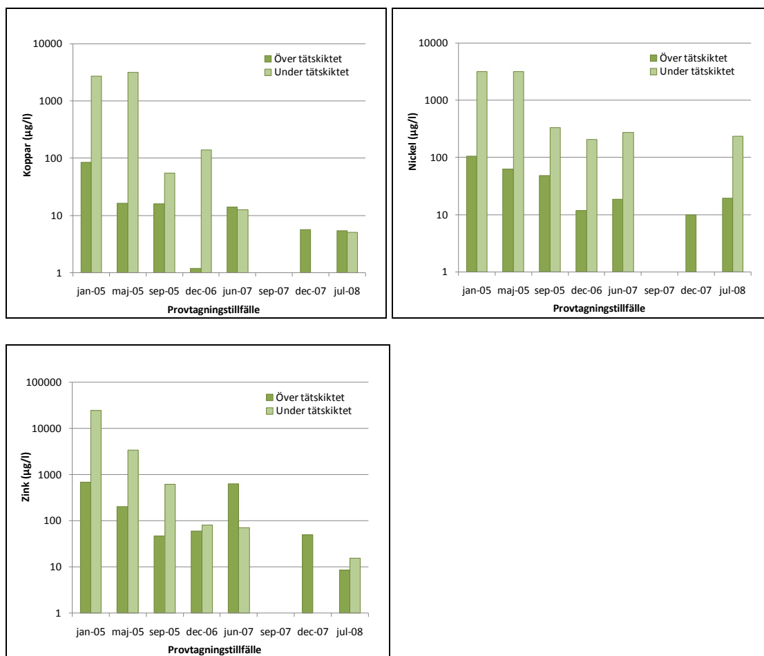
Figur 2-6 Halter av koppar, nickel och zink i vatten från lysimetrar och avrinningsytor i provytan på Gärstad. Medelvärde har beräknats för provtagningspunkter över respektive under tätskiktet. Observera att skalan på y-axeln är logaritmisk.
