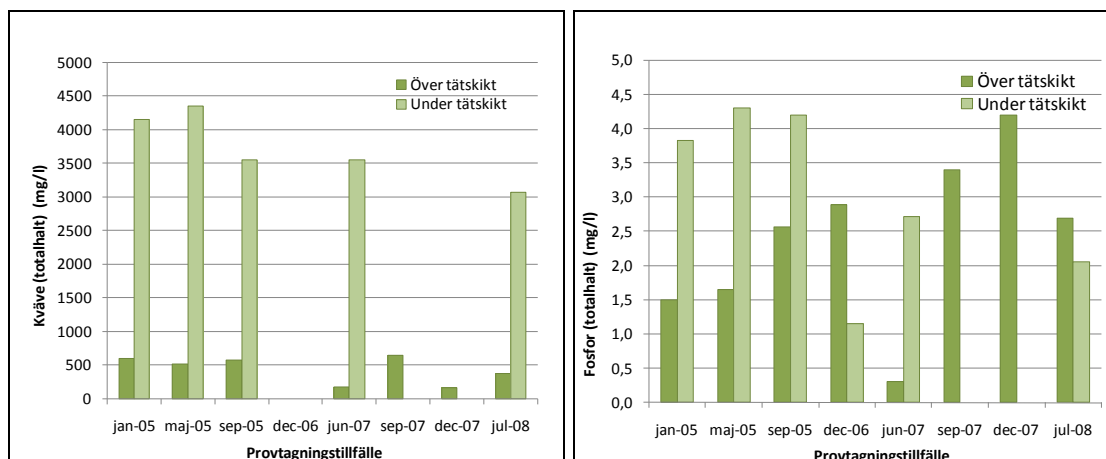
Figur 2-4 Kväve- och fosforhalter i vatten från lysimetrar och avrinningsytor i provytan på Gärstad. Medelvärde har beräknats för provtagningspunkter över respektive under tätskiktet.
