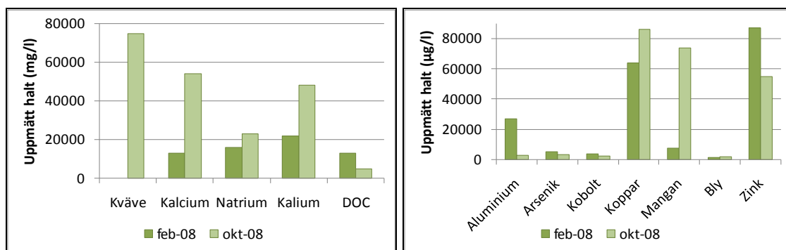
Figur 2-1 Uppmätta halter av näringsämnen, organiskt kol och grundämnena i prov från lysimeter under tätskiktet på den flacka delytan, Sofielund.
