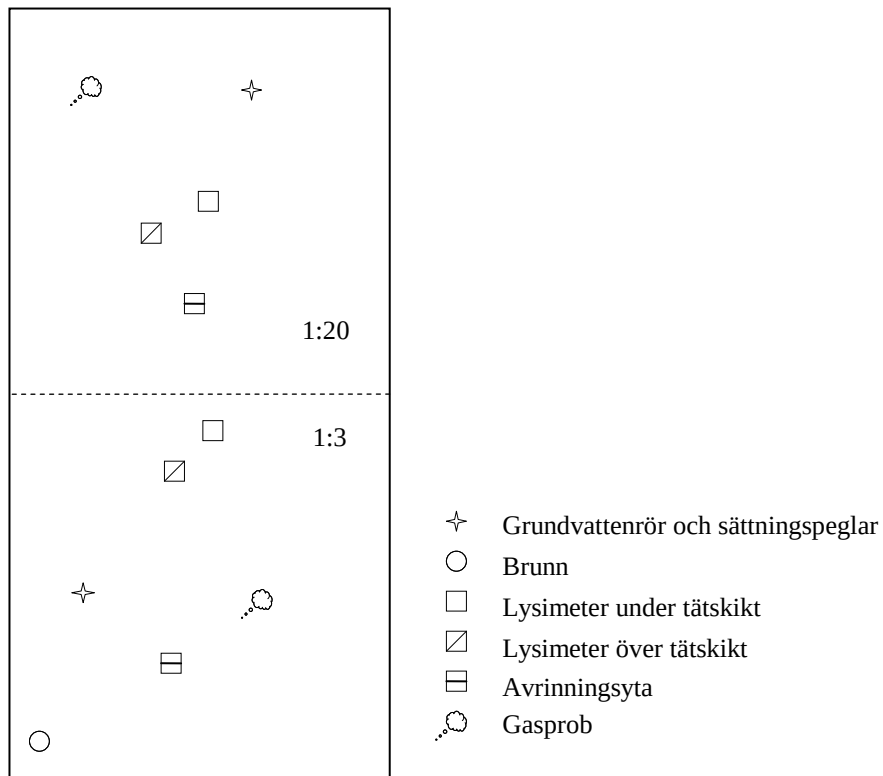
Figur 1-2 Översiktlig skiss (ej skalenlig) över provyta med installationer på SRV återvinnings anläggning, Sofielund. Lysimetern under tätskiktet på den branta delytan, sitter ganska långt upp i sluttningen, vilket gör att vattnet till denna inte har passerat så mycket material som det hade kunnat göra om lysimetern suttit längre ner.
