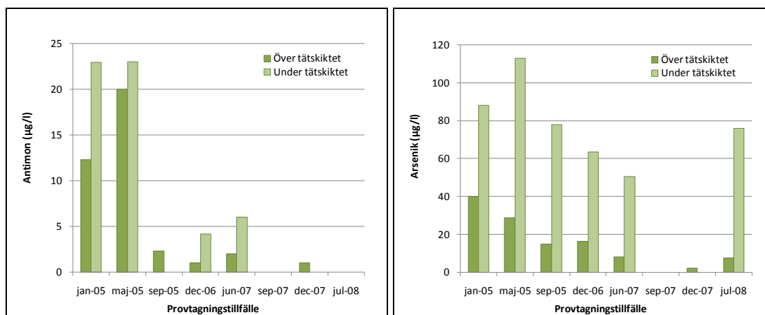
Figur 2-7 Halter av antimon och arsenik i vatten från lysimetrar och avrinningsytor i provytan på Gärstad. Medelvärde har beräknats för provtagningspunkter över respektive under tätskiktet.
