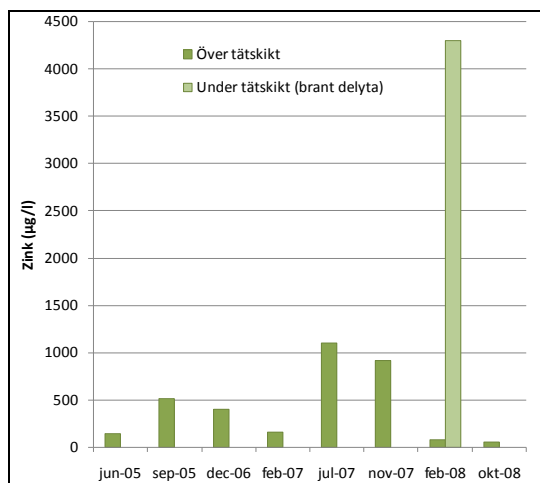
Figur 2-2 Uppmätta zinkhalter för lysimetrar och avrinningsytor på Sofielund. Värdet över tätskikt är beräknade som medel för avrinningsytor och lysimetrar ovan tätskiktet. Värdet för "under tätskikt" är resultat för lysimetern under tätskiktet på den branta delytan.
